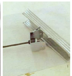
Modo de fallo. Rotura de las guías del perfil.
